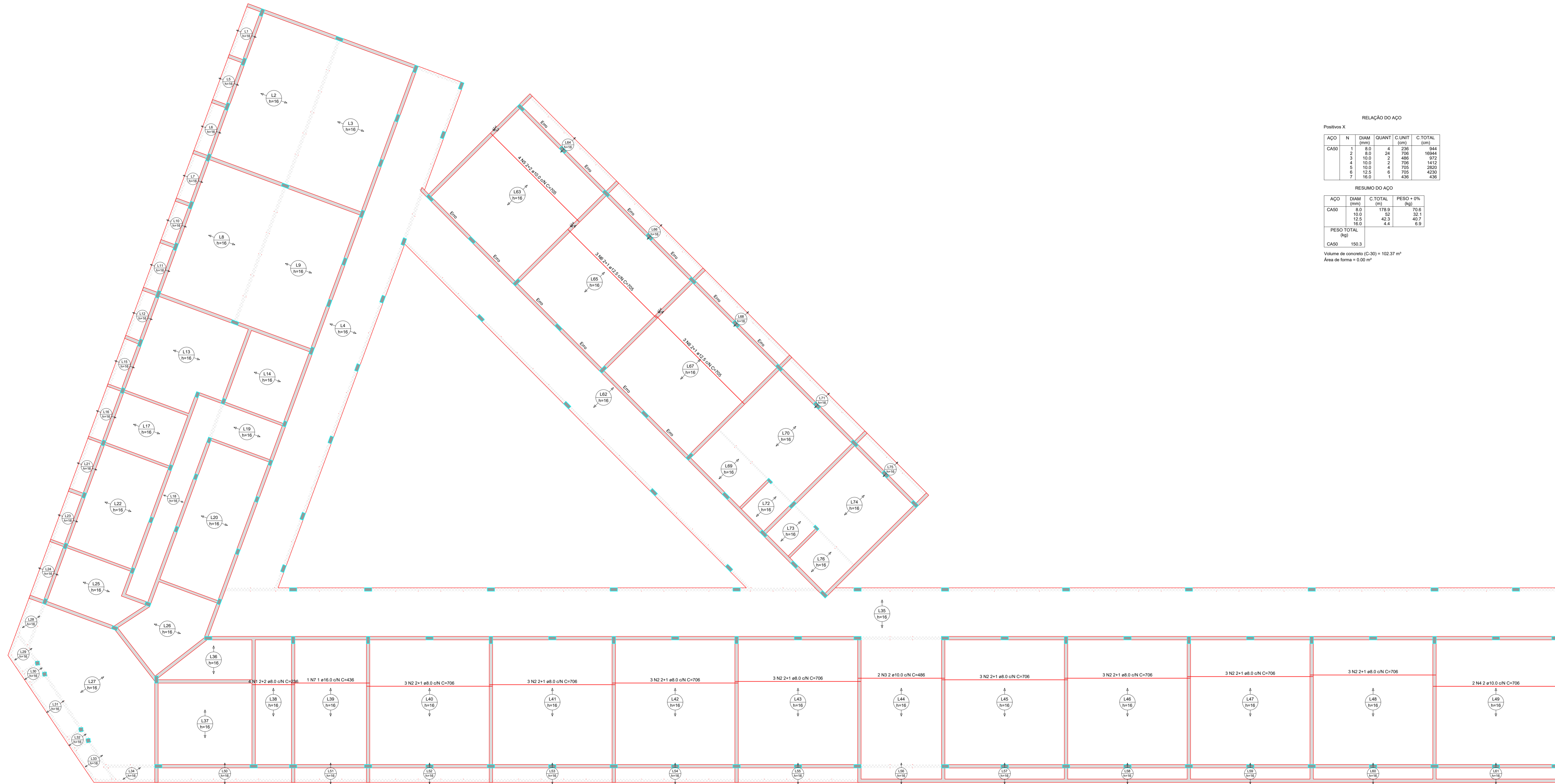
ARMAÇÃO POSITIVA DAS LAJES DO PAVIMENTO COBERTURA (EIXO X) escala 1:100
