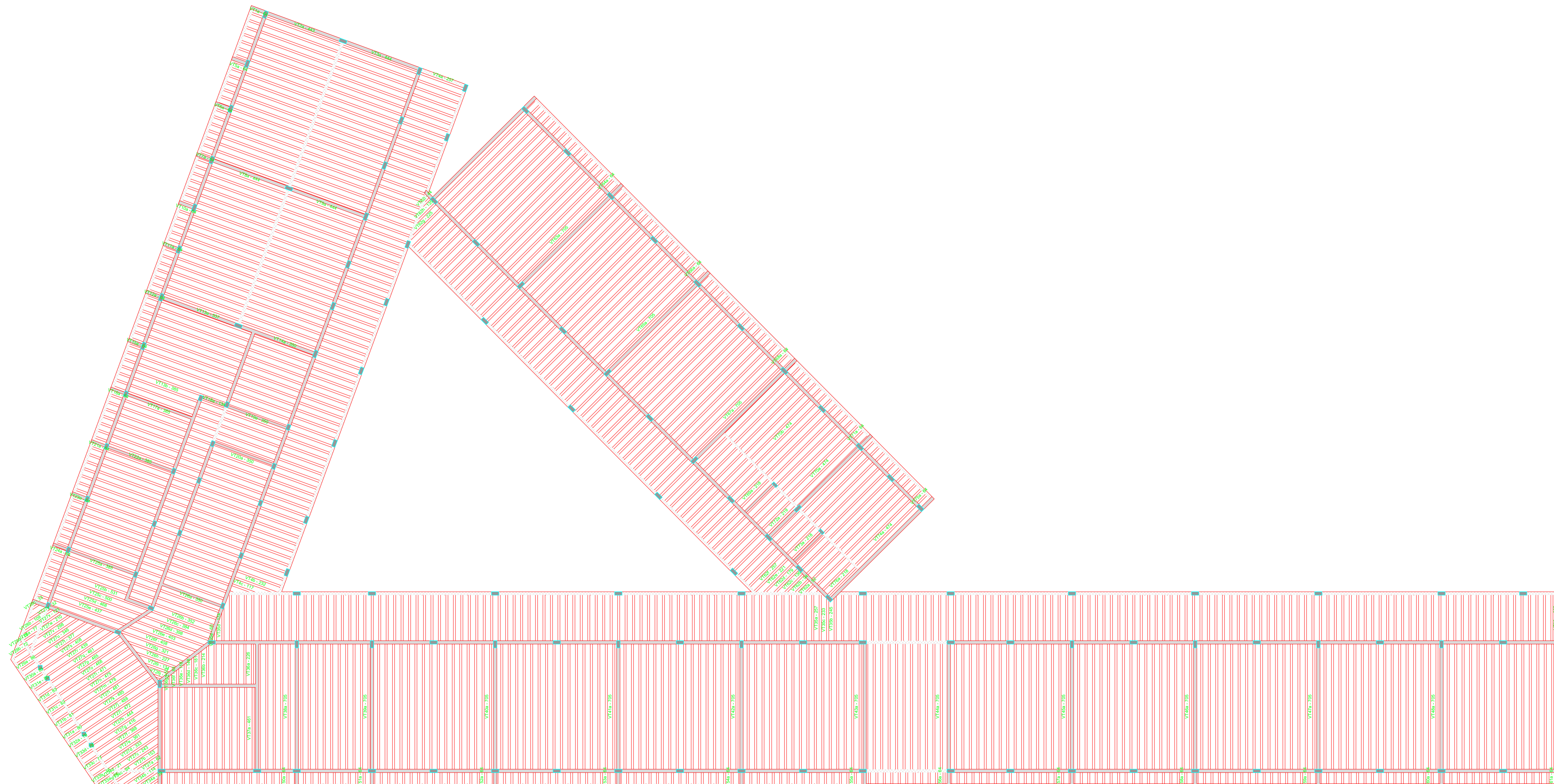
PLANTA DE VIGOTAS PRÉ-MOLDADAS escala 1:100
